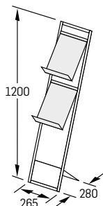
P-2 2 DIN A4-Acryl- Ablagen
