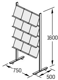
P-12 12 DIN A4-Acryl- Ablagen, fahrbar
