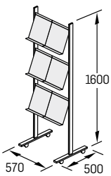
P-6 6 DIN A4-Acryl- Ablagen, fahrbar
