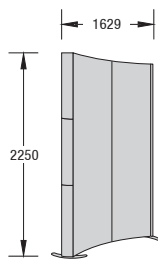
VA 5823 P1 für 2 Paneele seitliche Aluminium- profile, silber eloxiert, inkl. 1 Spot
