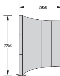
VA 5843 P1 für 4 Paneele seitliche Aluminium- profile, silber eloxiert, inkl. 2 Spots
