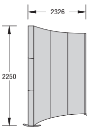
VA 5833 P1 für 3 Paneele seitliche Aluminium- profile, silber eloxiert, inkl. 2 Spots
