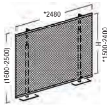
OP 100 Banner-Set gerade 2 Teleskopstützen und 4 Kederzargen 1240 mm lang, inkl. 2 Fußplatten
