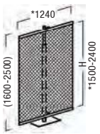
OP 10 Banner-Set gerade 1 Teleskopstütze und 2 Kederzargen 1240 mm lang, inkl. 1 Fußplatte
