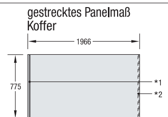
*1 VA 5035 Magnetband (Vorderansicht)
