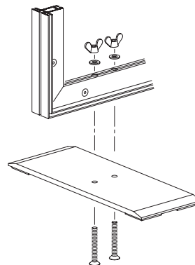
M 1347 Grundplatte
