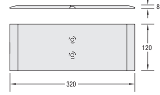
M 1347 Grundplatte Stahl
